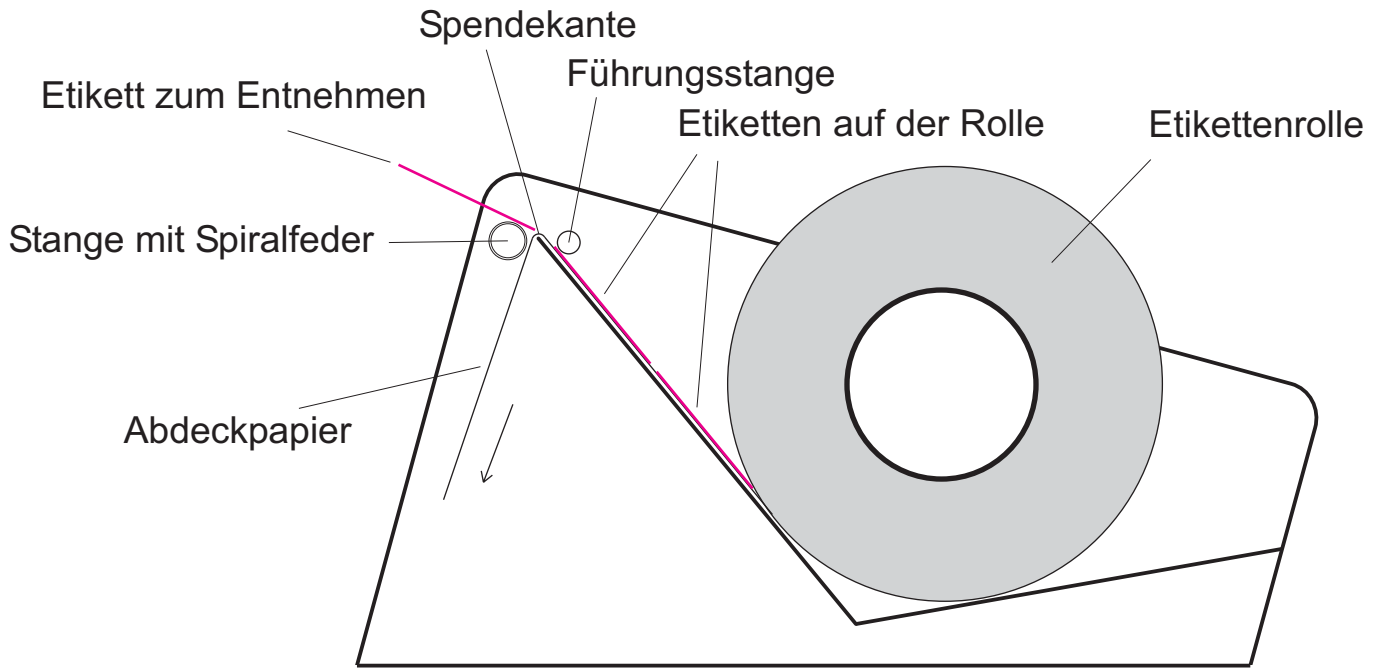
Etikettenspender in der Seitenansicht
